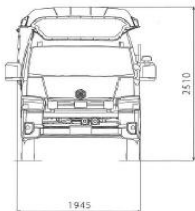
寸法図 単位 (mm)
