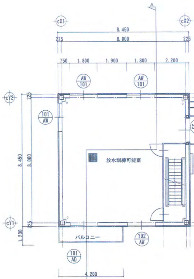
5階平面図 S=1/100
