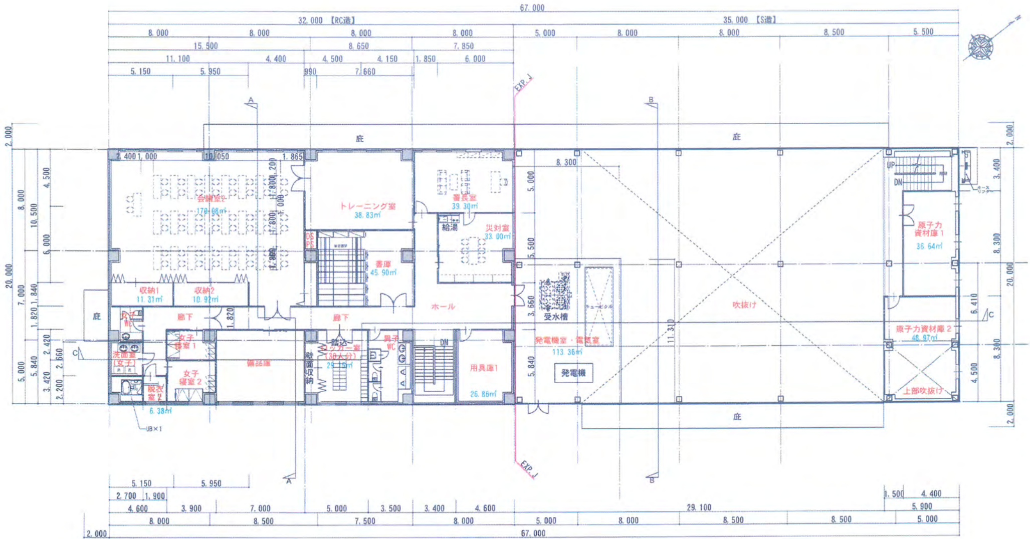
2階平面計画図 S=1/200 ※窓は打合せにより決定することとする。
